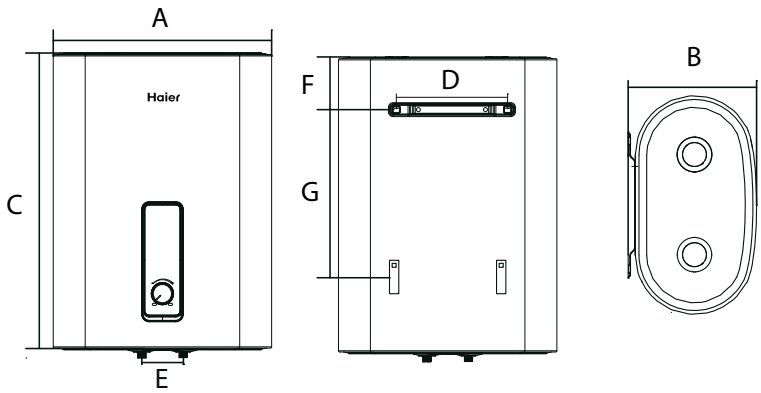
Габаритные размеры (мм)
